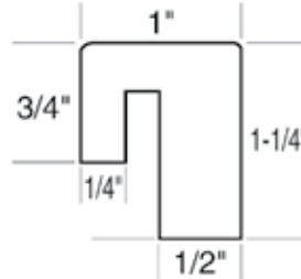
T-564-JS-2 19" OD x 1" CS
