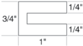
#22-B-945 15-3/4" ID x 17-3/4" OD
