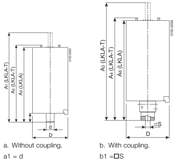
Fig. 2. Dimensions - actuator.
