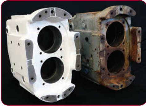
GEARCASE
